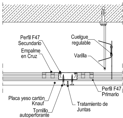
Tratamiento de juntas cantos vivos
