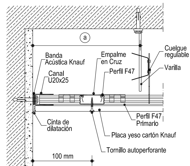
Encuentro con muro
